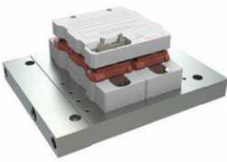
SKiiP® 3
